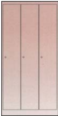
MOS-31K 3人用 W900xD515xH1790 單格W267xD476xH1628
