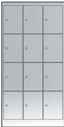
MOS-34K 12人用 W900xD515xH1790 單格W267xD476xH392
