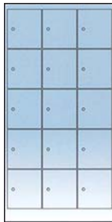
MOS-35K 15人用 W900xD515xH1790 單格W267xD476xH298
