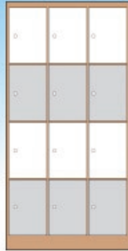
外部尺寸 12人用 W900×D475×H1870 單格 W267×D438×H392 重量：65kg
