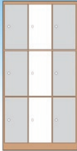
外部尺寸 9人用 W900×D475×H1870 單格 W267×D438×H533 重量：65kg
