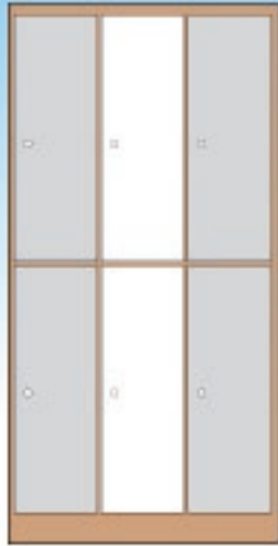
外部尺寸 6人用 W900×D630×H1870 單格 W267×D598×H812 重量：70kg
