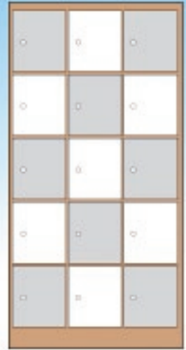
外部尺寸 15人用 W900×D475×H1870 單格 W267×D438×H310 重量：75kg
